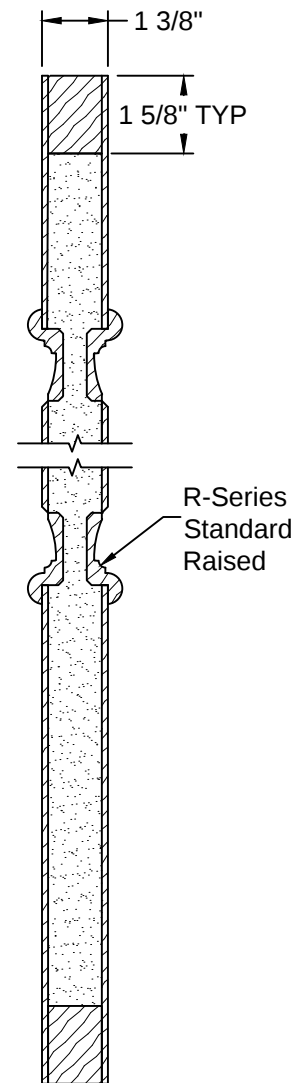
Section A-A
