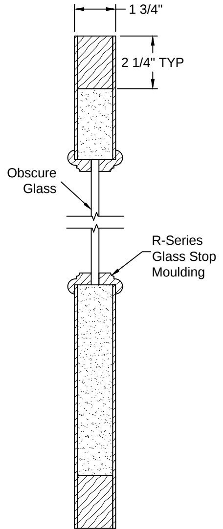
Section A-A
