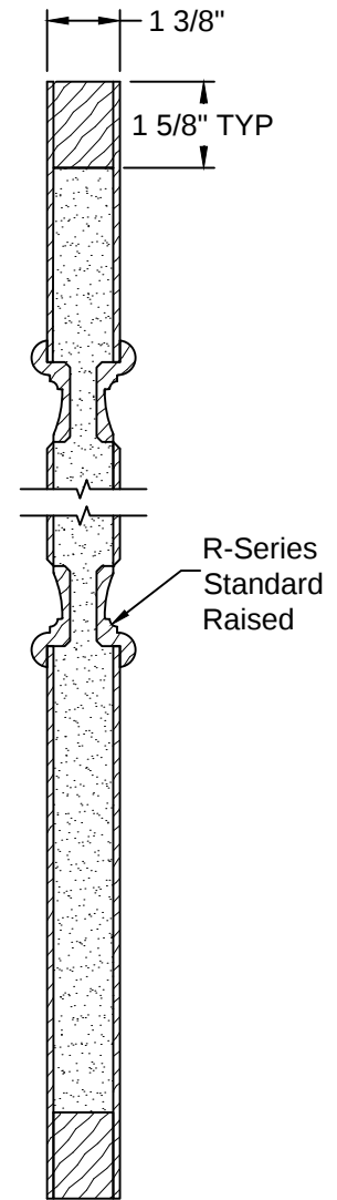
Section A-A
