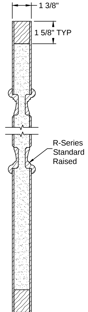
Section A-A
