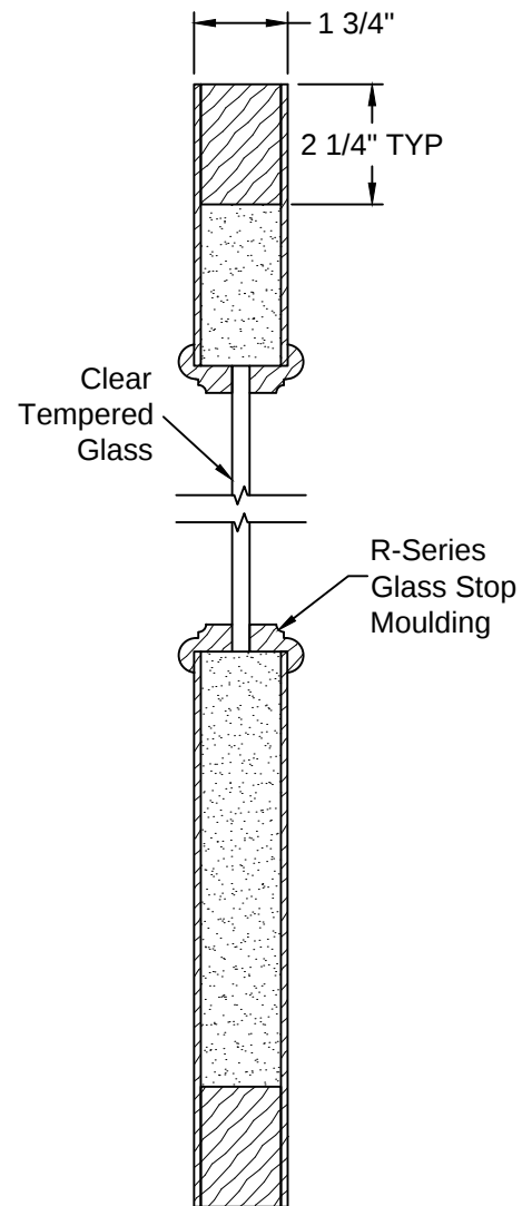
Section A-A
