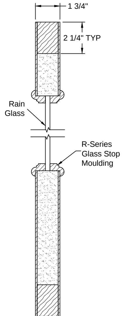
Section A-A
