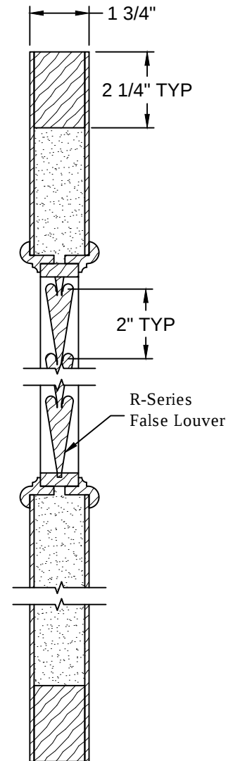
Section A-A
