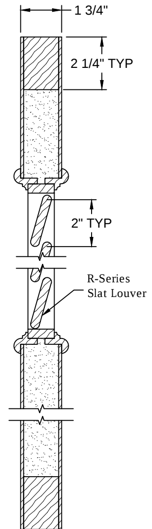
Section A-A
