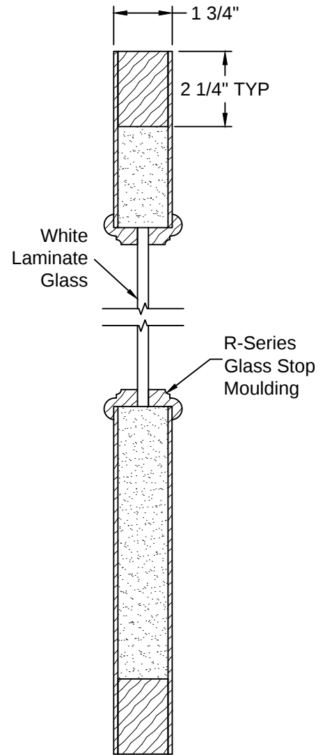
Section A-A
